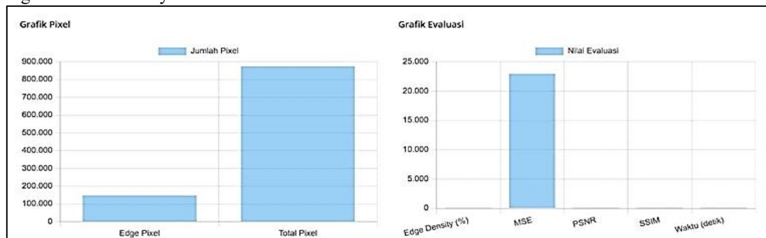
Gambar 21. Grafik Evaluasi Hasil Deteksi Tepi
